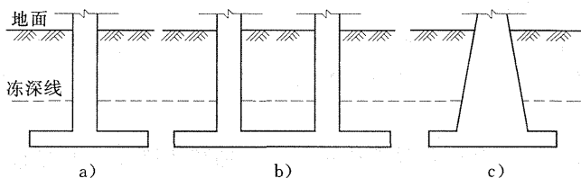
图5 基础型式示意图
