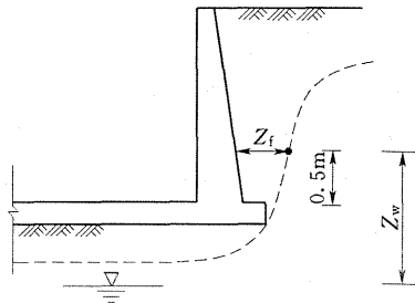
图 4 冻胀量 h_d 的计算点示意图
