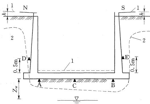
图 3 控制断面计算点、地基土设计冻深线、冻胀位移线示意图
