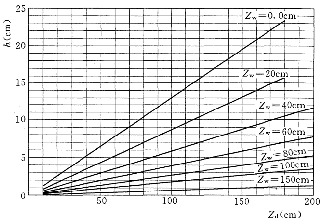
图 C.0.2-3 砂(砾)类土的冻胀量图
