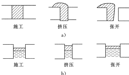
图 1 缝的构造示意图
