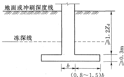
图 6 扩大式基础尺寸示意图
