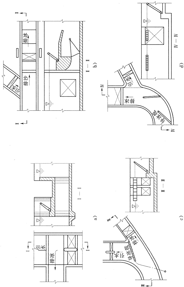
图 2 前池引水、排冰布置示意图
