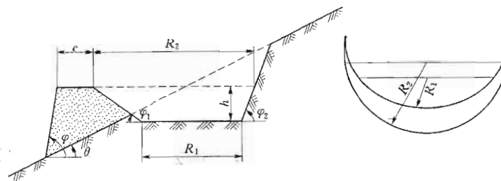
图6 鱼鳞坑整地示意图
