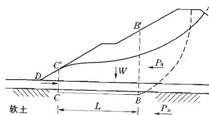
图 F.0.2 改良圆弧法计算简图
