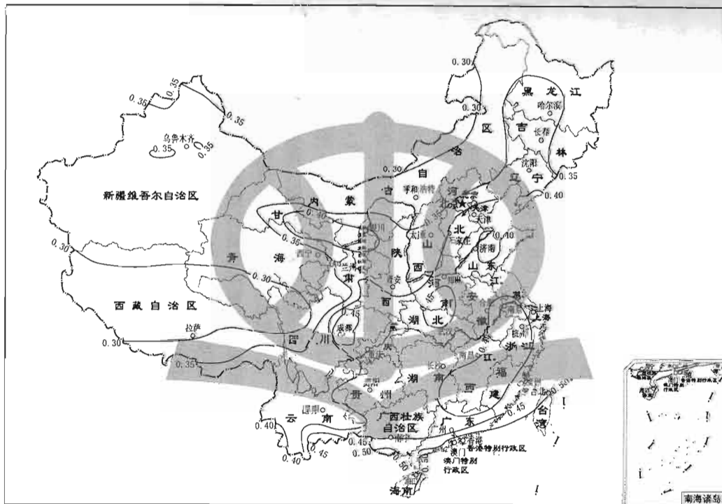
图 5.3.1-2 中国 60min 降雨强度转换系数 C_{60} 等值线图
