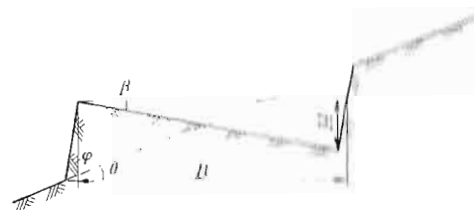
图5 反坡梯田示意图
