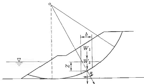
W 1 —在弃渣边坡外水位以上的条块重力; W 2 —在弃渣边坡外水位以下的条块重力
