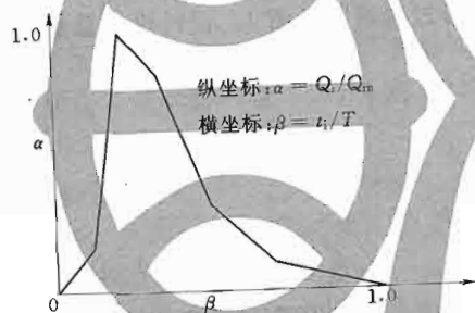
图3 无量纲过程线模型
