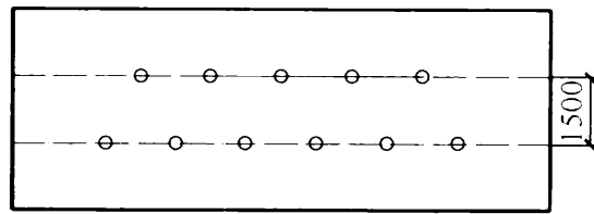
图 C.0.2-2 双层布置图
