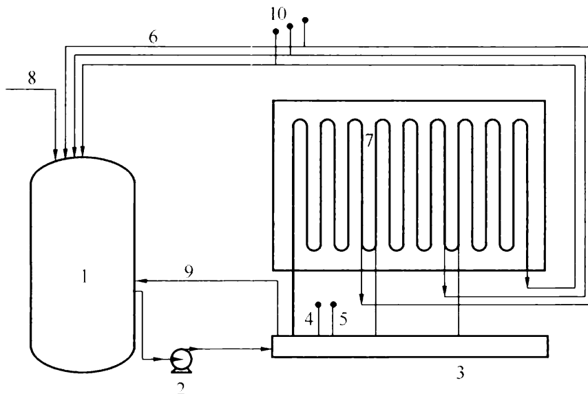
图 C.0.3 水冷却系统图
