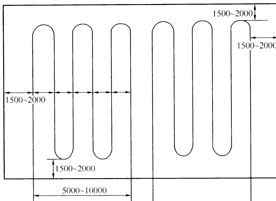
图 C.0.1 冷却水管平面布置图
